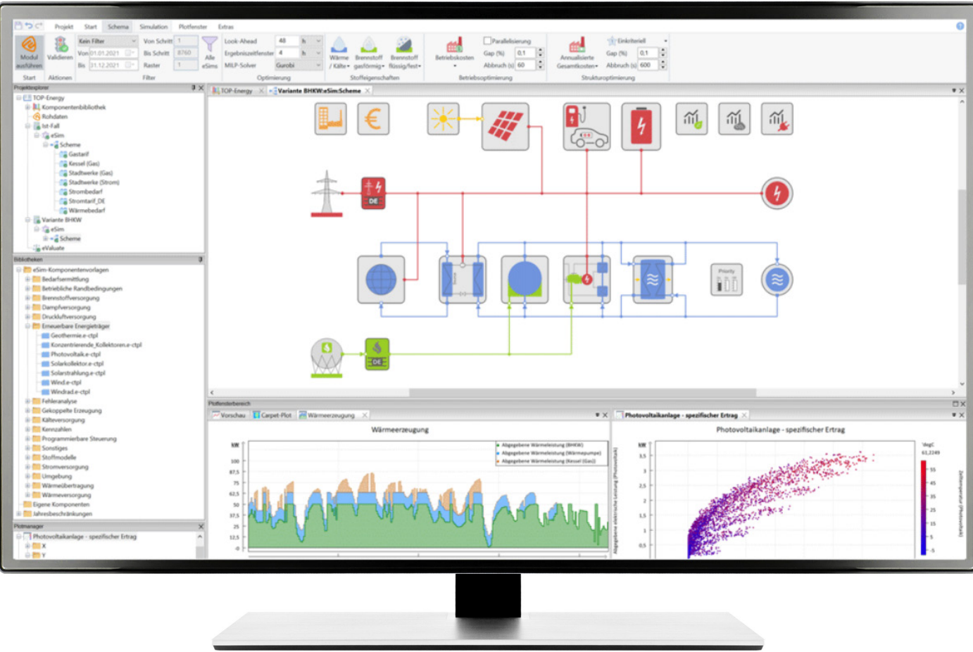
Potenzialanalyse - Einbindung von Stromspeicher und PV im Gebäude-Energiesystem
