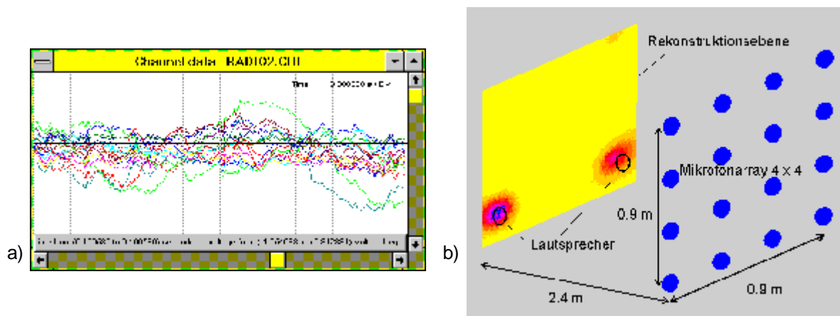
Fig. 4: Geräuschkarte eines Stereoradios. Kanaldaten a) und Versuchsaufbau mit berechneter Erregungskartierung b)
