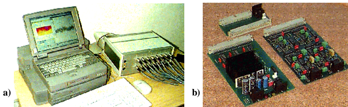
Fig. 11: a) Entwickler Meßplatz, bestehend aus Laptop mit Dockingstation und Vorverstärker (rechts) b) Speziell entwickelte Leiterkarten des Vorverstärkers
