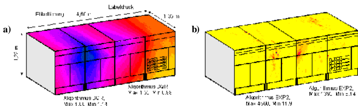
Fig. 5: Erste Schallkartierungen mit PSI-Tools: Schallemissionsbild an einer Briefetikettiermaschine 1) : a) integraler Schall (höchste Leistung) b) Spitzenemission (höchste Energie), Farben: max. blau, min. gelb Aufnahmedauer 3 Sekunden
