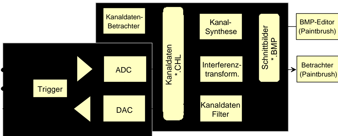
Fig. 10: Vermaschung von Soft- und Hardware beim PSI-Messplatz. Es ist möglich, Kanaldaten in Erregungskarten umzurechnen. Zu Testzwecken steht eine inverse Funktion zur Verfügung.
