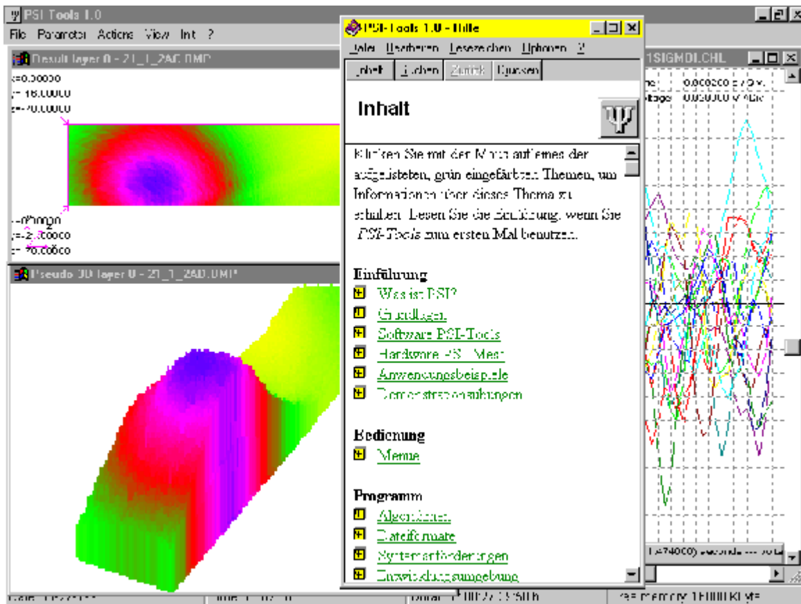
Fig. 12: Oberfläche PSI-Tools. Aufnahme eines PKW in 70 Metern Entfernung. In der Mitte ist der geöffnete Help-File zu erkennen; rechts sind die Kanaldaten zu erkennen, aus denen der PKW-Ort (links) berechnet wurde (Windows'95/Windows for Workgroups 3.11)
