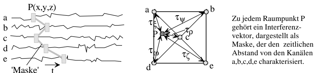
Fig. 3: Prinzip der Interferenztransformation. Jeder Raumpunkt P besitzt eine typische Maske in den Kanaldaten, über die das Vorhandensein einer Erregung an diesem Punkt festgestellt werden kann
