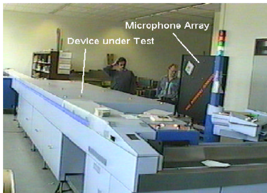
Fig. 6: Zugehöriger Versuchsaufbau. Im Vordergrund ist die (geschlossene!) Briefetikettiermaschine zu erkennen, im Hintergrund rechts steht das 16-Kanal-Mikrofonarray (schwarz) mit dem Meßplatz
