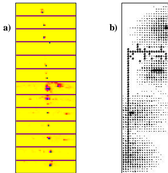
Fig. 8: Kurzzeitintegrale. Die Bildserien sind schlüssig über je eine zehntel Sekunde entwickelt, Algorithmus MULT a) Ford Fiesta auf der Kekulestraße. Deutlich ist die Erregungspur von links nach rechts zu erkennen. Bildausschnitt 50 x 10 Meter; b) Bus in einer Entfernung von 170 Metern: Bildausschnitt 6x5 Meter
